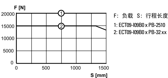
柱负载限制与行程
