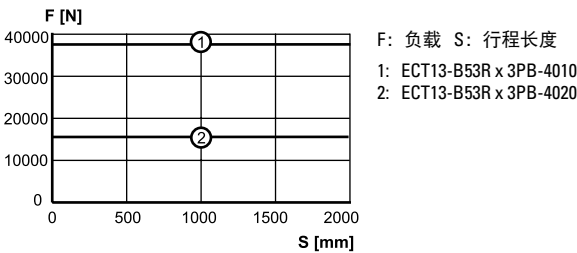
柱负载限制与行程
